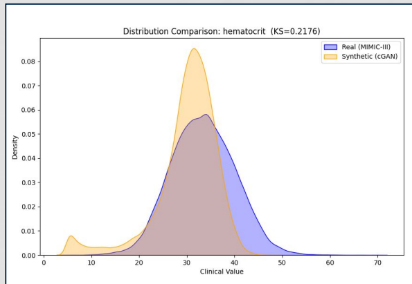
GAN
